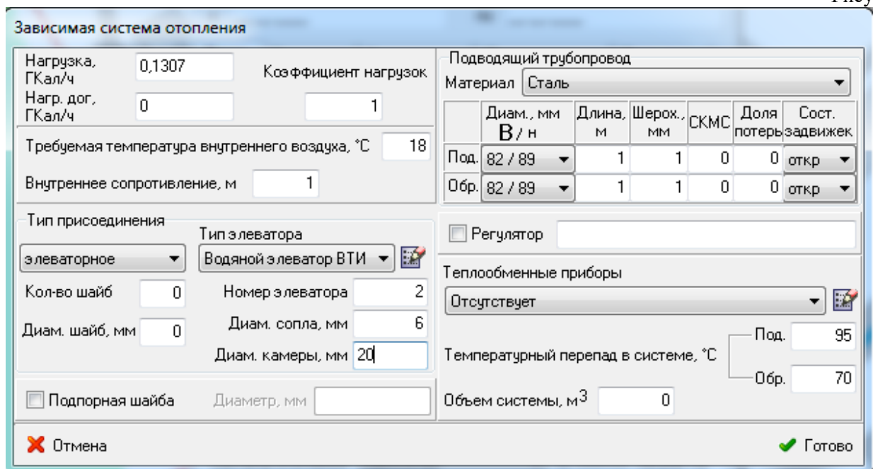
Паспортизация участка тепловой сети тепловой энергии
